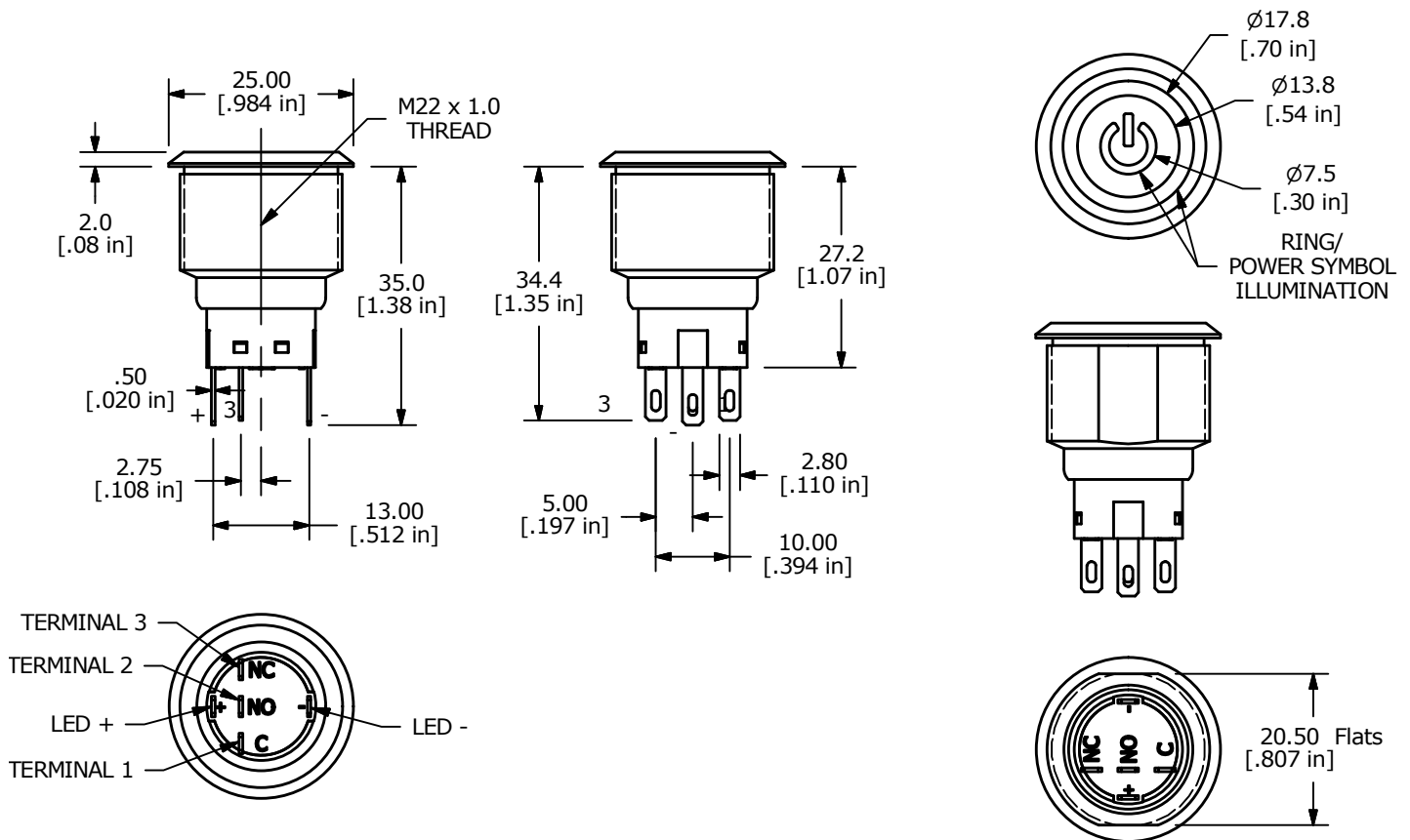
SPDT SWITCH DIMENSIONS
